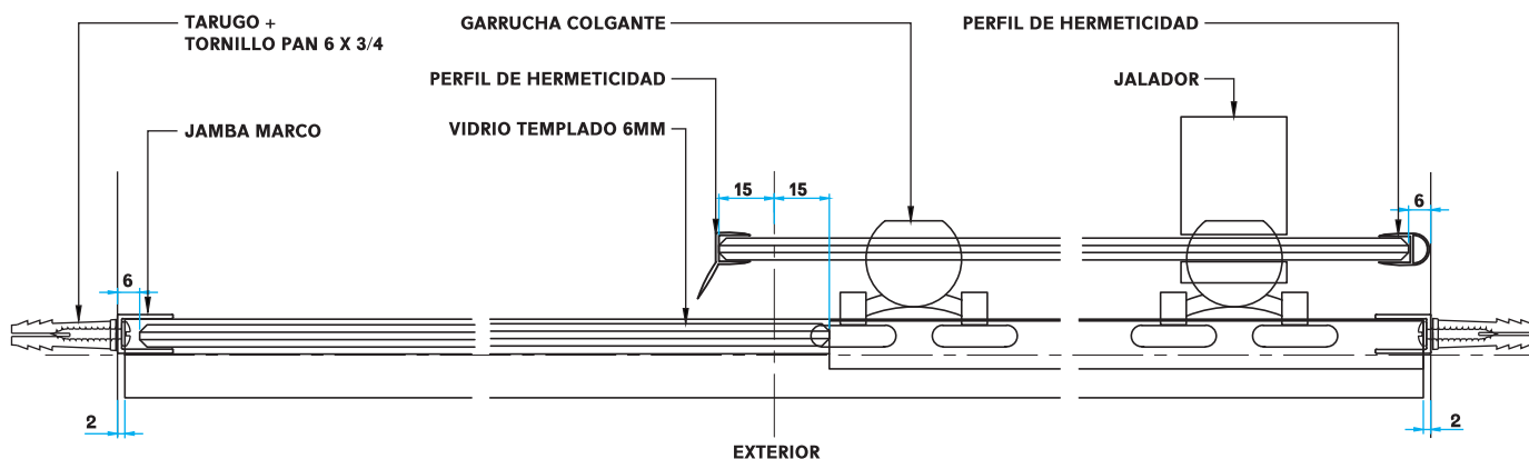
CORTE 3-3
